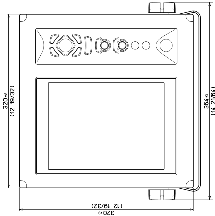
Front view 正面図
